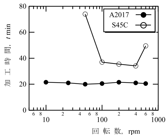
図2. 各回転数における加工時間
