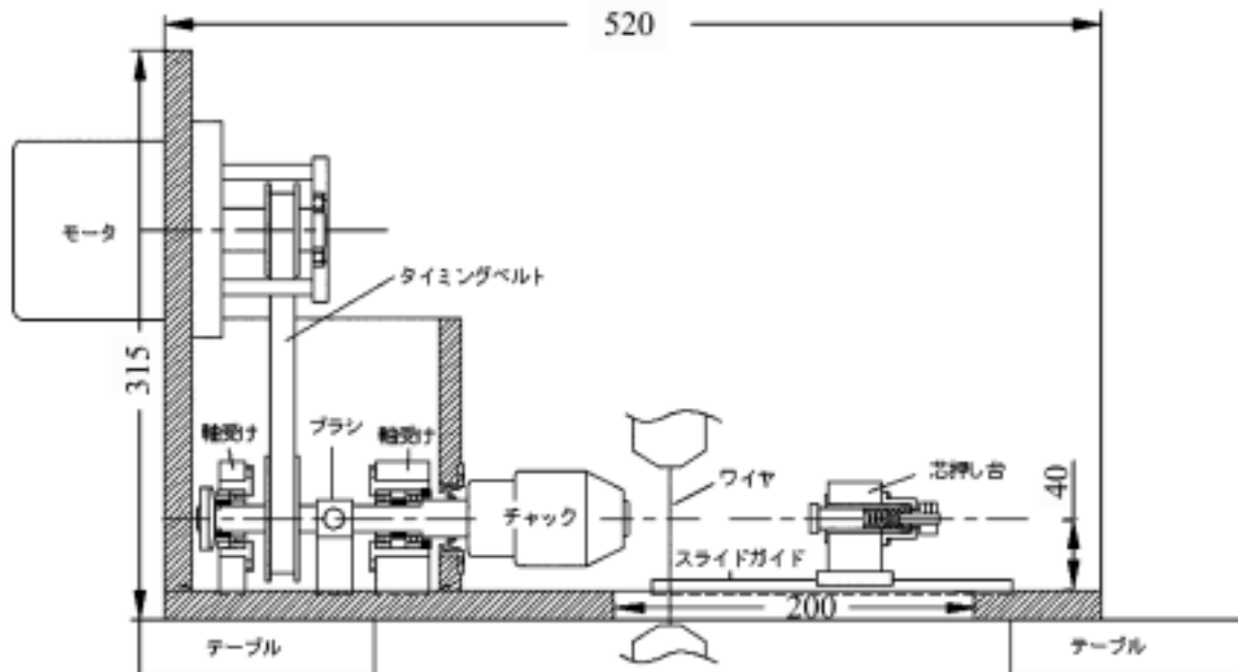
図 1. 旋削装置の概観
