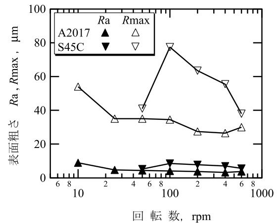
図5. 各回転数における加工表面の粗さ
